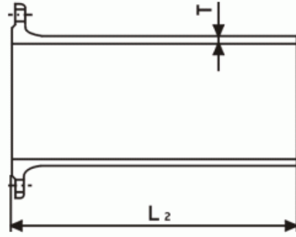
■ 短管2號 Flanged Spigot
