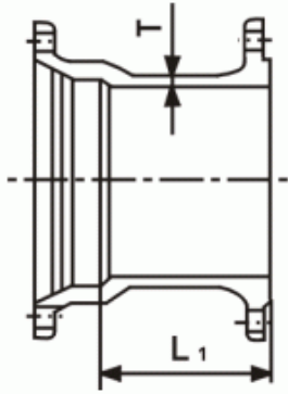
■ 短管1號 Flanged Socket
